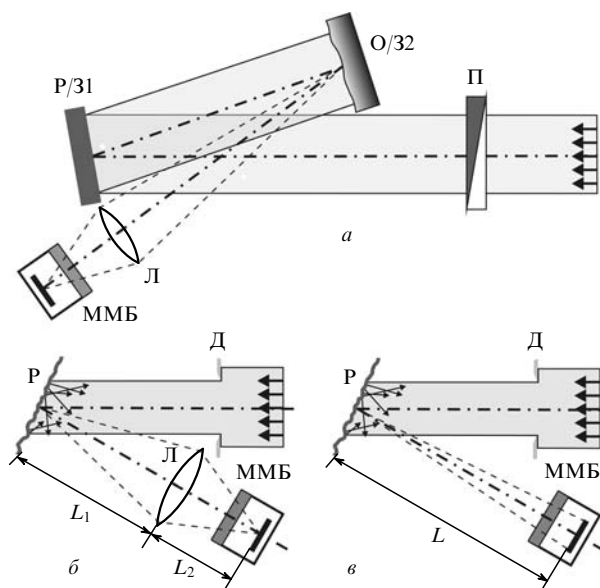
Рис. 1. Схема установки для записи изображений в терагерцевом диапазоне (а) и ее модификации для исследования субъективных (регистрация через линзу) (б) и объективных (непосредственная регистрация) (в) спеклов:
